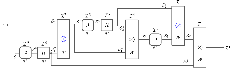
Fig. 6: AES \cdot^{254}
