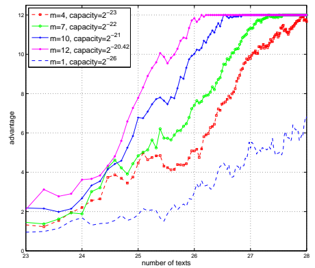
(d) Empirical advantage for LLR-method
